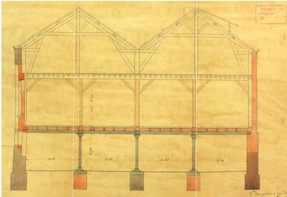
Figuur 4. Het houten pakhuis op de Werfkaai heeft een houten structuur op de verhoogde begane grond en op zolderniveau. De structuur in de kelder bestaat uit gewelfde bakstenen vloeren ondersteund door ijzeren balken en gietijzeren kolommen. Werfkaai 3.
