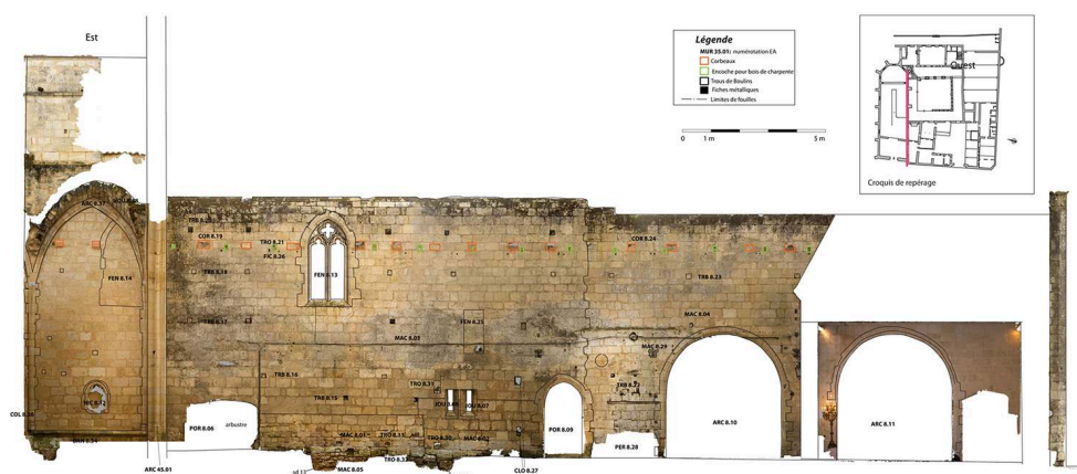
Fig. 3 – Analyse du bâti du mur intérieur sud de l'église
