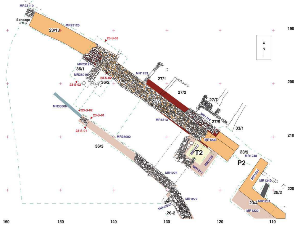
Fig. n°3 : Plan de détail de la porte récente (P2) flanquée une tour carrée à noyau de terre (T2), ainsi que de la courtine sud-ouest de l'enceinte et des avant-murs.
