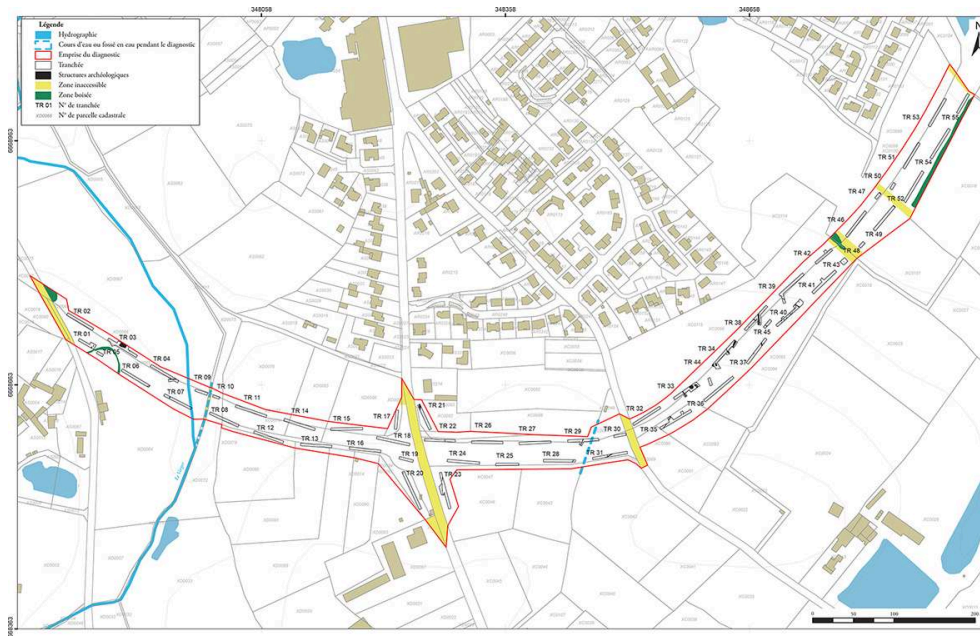
Fig. 1 – Plan général de l'opération
