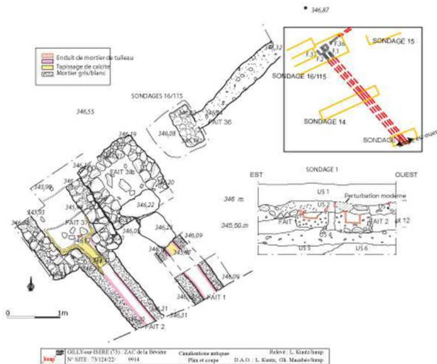
Fig. n°1 : Canalisations antiques - Plan et coupe
