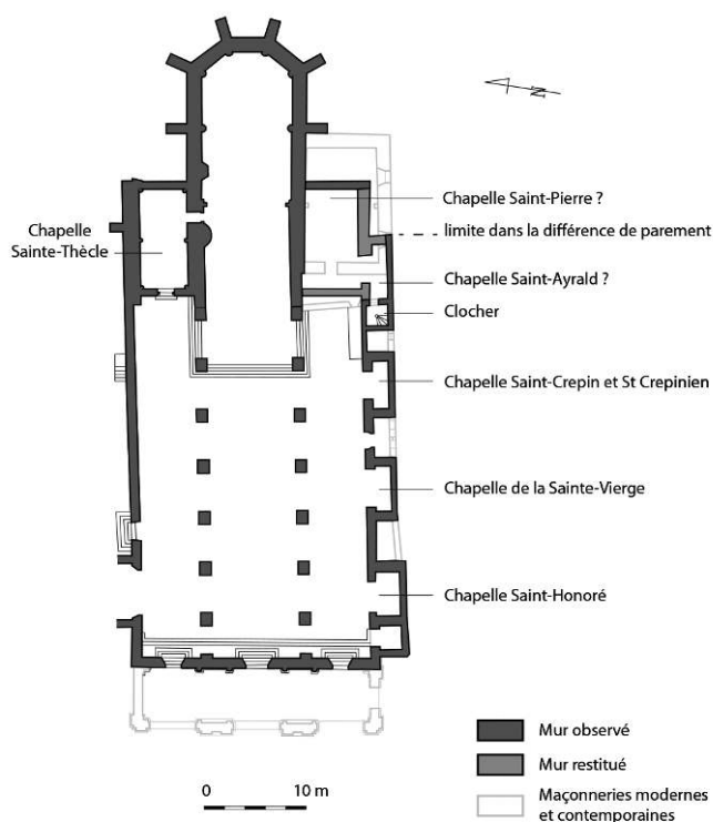
Fig. 1 – Plan de la cathédrale
