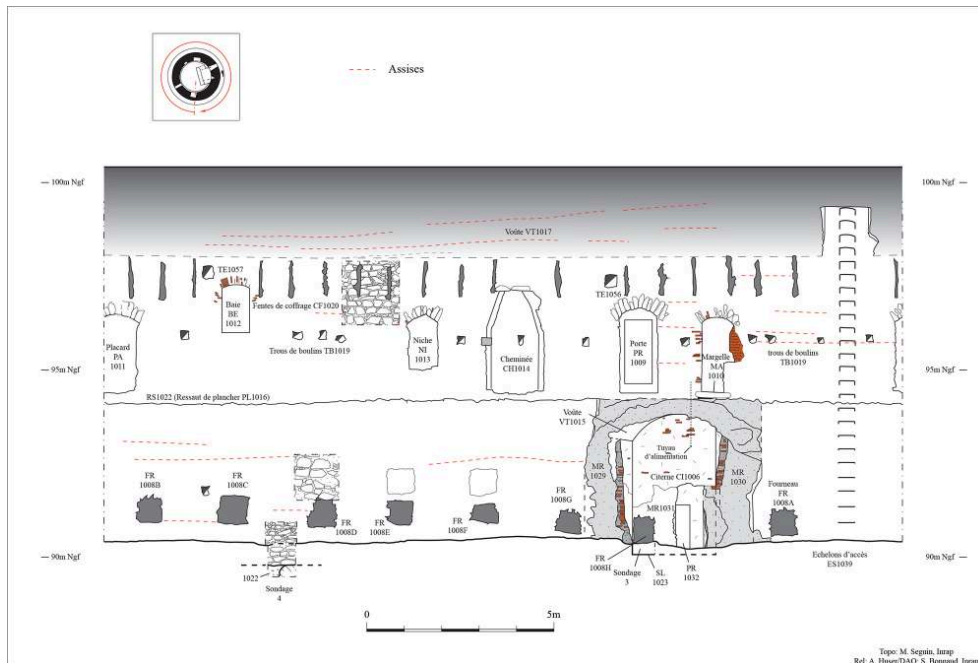
Fig. 2 – Traduction graphique du développé intérieur de la tour de la Castagna
