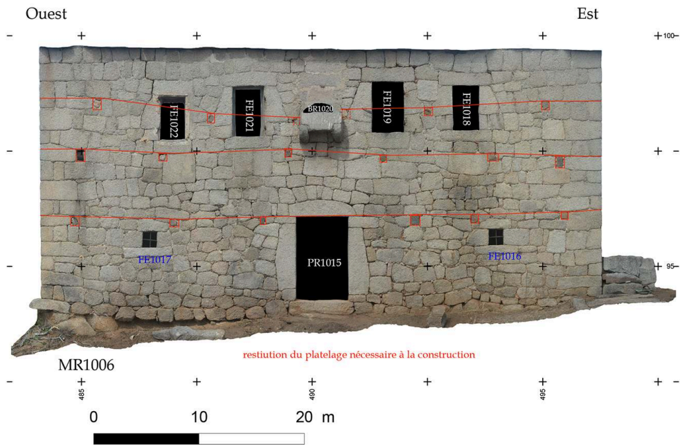
Fig. 2 – Mur de façade sud équipé de sa bretèche
