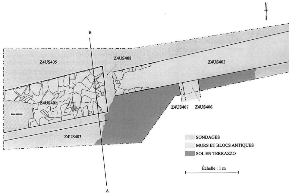
Fig. 2 – Plan du sondage n° 5, situé dans la cave n° 4
