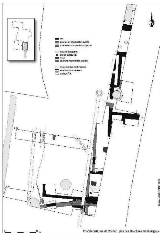
Fig. n°1 : Plan des structures
