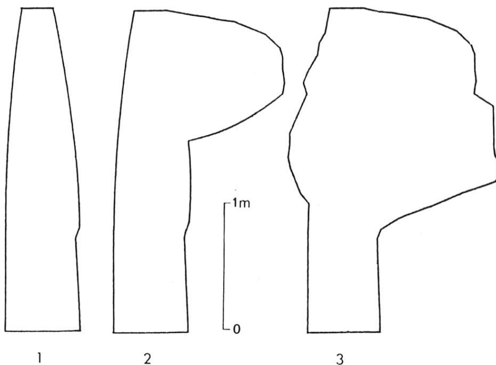
Fig. 1 – Auxelles-Haut, mine Saint-Jean, section 6 du travers-banc à la cote 600
