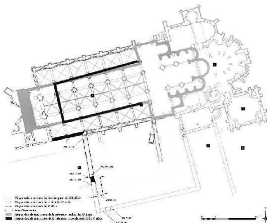
Fig. n°2 : Plan masse et proposition de restitution aux X e s., XI e s. et XII e s.
