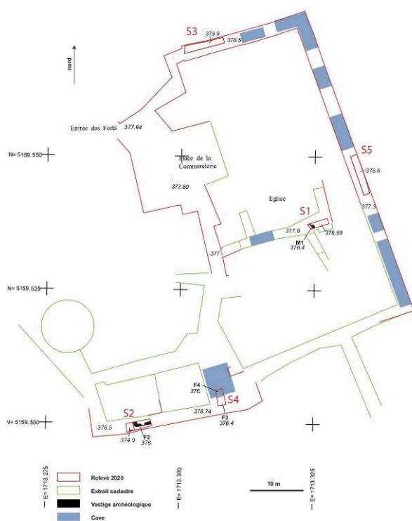
Fig. 1 – Plan topographique des sondages
