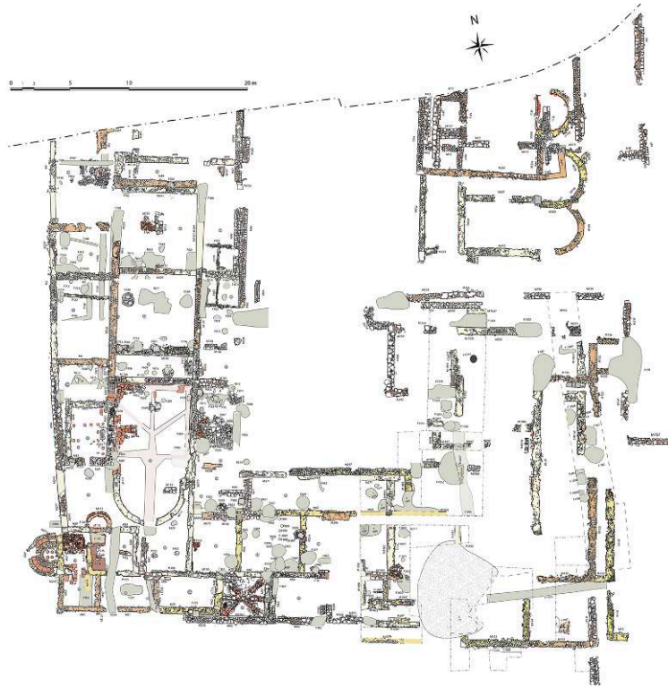
Fig. 1 – Plan des vestiges de l'angle sud-est du bâtiment résidentiel de la villa gallo-romaine de Saint-Saturnin-du-Bois
