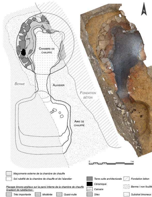
Fig. 1 – Plan et orthophotogrammètrie du four de potier
