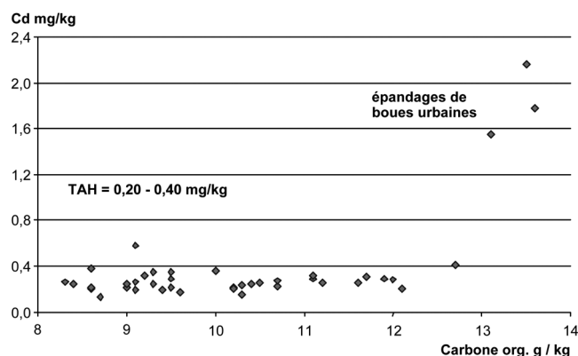
Figure 1 : Illustration de la notion de « teneur agricole habituelle » (TAH). Exemple de 39 horizons labourés de Néoluvisols issus de loess du Vexin français. On notera l'absence de relation entre les teneurs en cadmium et l'abondance du carbone organique. Les horizons de surface labourés de ce type de sol, quelle que soit leur teneur en carbone, présentent des teneurs agricoles habituelles en cadmium comprises entre 0,20 et 0,40 mg/kg. Les trois valeurs beaucoup plus élevées correspondent à des contaminations par des épandages massifs de boues urbaines réalisées dans les années 70. Figure 1: Illustration of the notion of usual agricultural content (UAC). The example of 39 ploughed horizons from Néoluvisols developed in loess (Vexin). There is no relationship between the cadmium contents and the abundance of organic carbon. The surface horizons of this soil type, whatever their carbon content, show cadmium UAC comprised between 0.20 and 0.40 mg/kg. The three particular values much higher correspond to contaminations by heavy spreading of urban sewage sludge made during the seventies.
