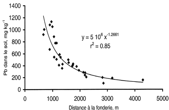
Figure 4 : Concentrations en plomb dans les horizons de surface des sols en fonction de la distance à la fonderie de Noyelles-Godault (Sterckeman et al. , 2000).
