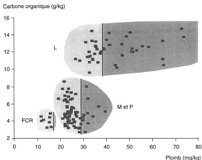
Figure 2 : Relation carbone organique/teneurs en plomb pour trois catégories d'horizons prélevés à proximité d'usines traitant du plomb (Baize, 2002). L = horizons de surface labourés. M et P = horizons de moyenne profondeur (40 à 60 cm) ou profonds (> 70 cm). FCR = matériau parental calcaire.
