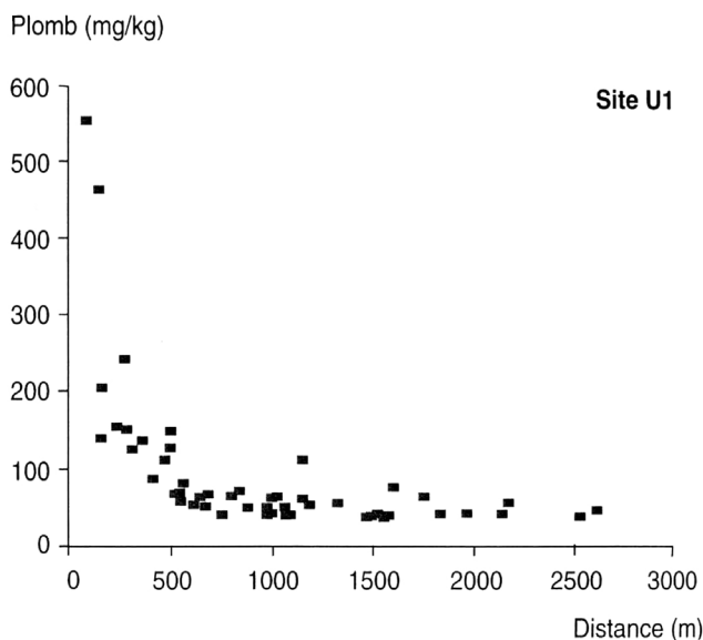
Figure 3 : Concentrations en plomb dans les horizons de surface en fonction de la distance à l'usine la plus proche (Beauce) (Baize, 2002).
