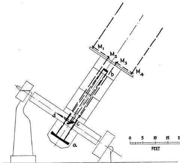
Figure 4 : Schéma de l'appareillage utilisé par Michelson et Pease au télescope de 2,50 m de diamètre du Mont Wilson pour mesurer le diamètre de Bételgeuse.
