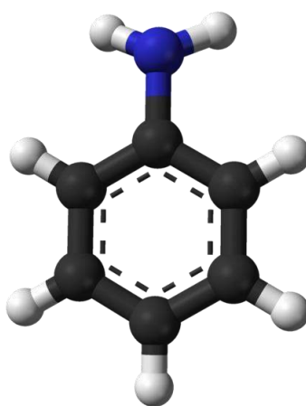
Figure 4 : Formule développée de l'aniline C_6H_5NH_2 . L'aniline a permis la découverte du premier colorant industriel, la mauvéine, par Perkin en 1858. Elle est à la base de la chimie des colorants, ainsi que produit de départ de la synthèse de nombreux médicaments.
