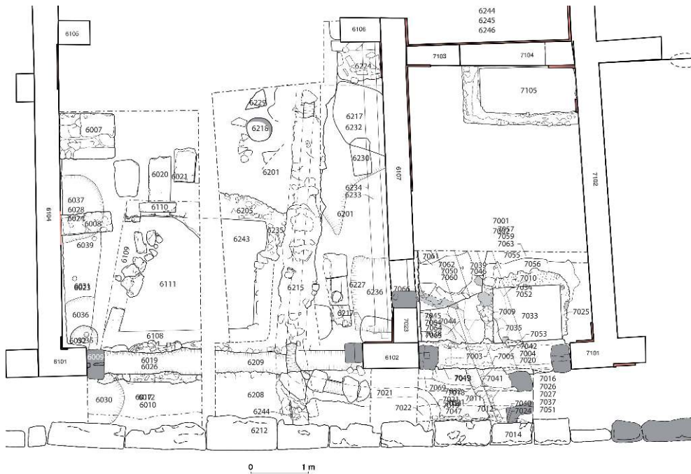
Fig. 1 - Pompéi. Plan de la boutique.
