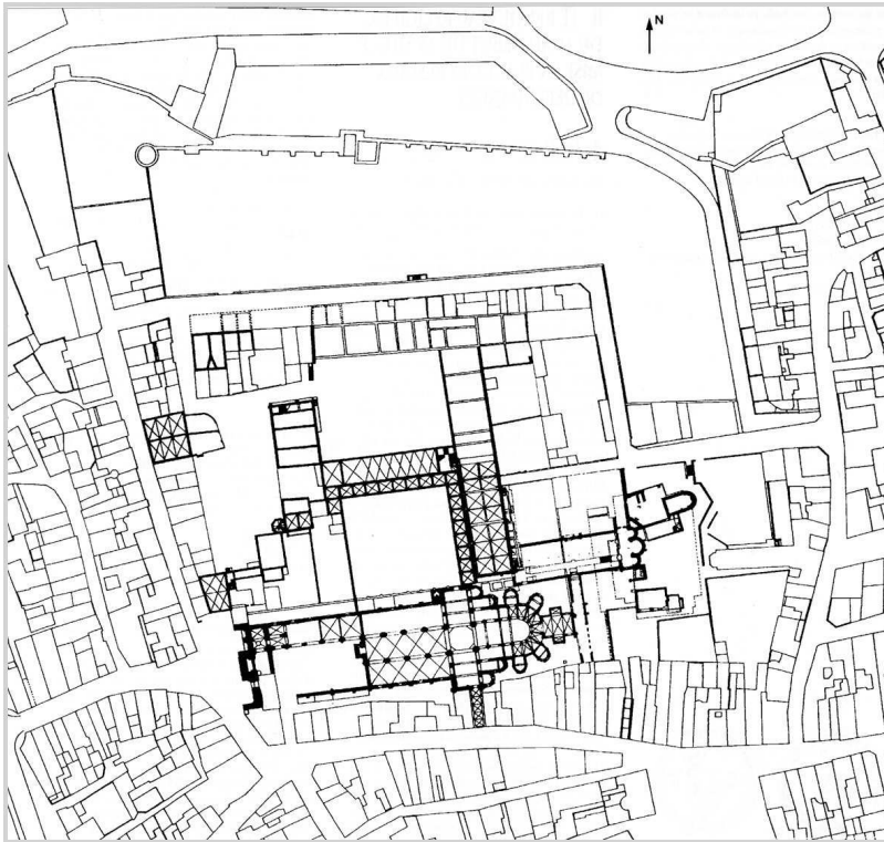
Fig. 1 - Plan du prieuré de La Charité-sur-Loire.
