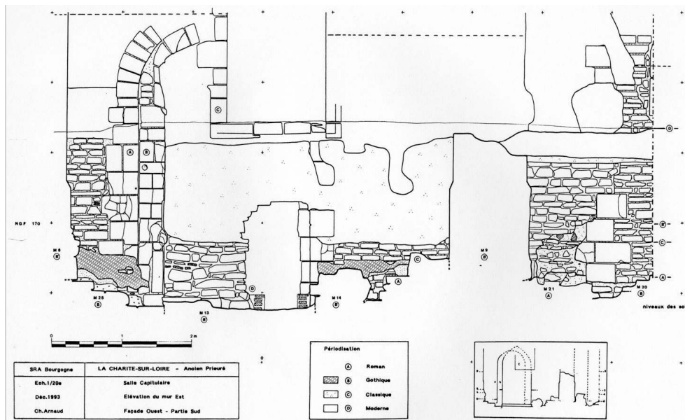
Fig. 2 – Élévation extérieure du mur est de la salle du chapitre (Ch. Arnaud).
