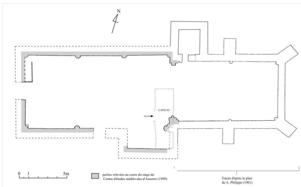
Crain, plan de l'église (dessin CEM).
