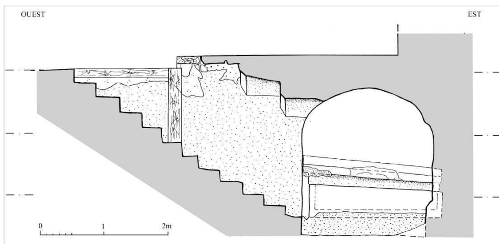
Crain, caveau en coupe (dessin CEM).
