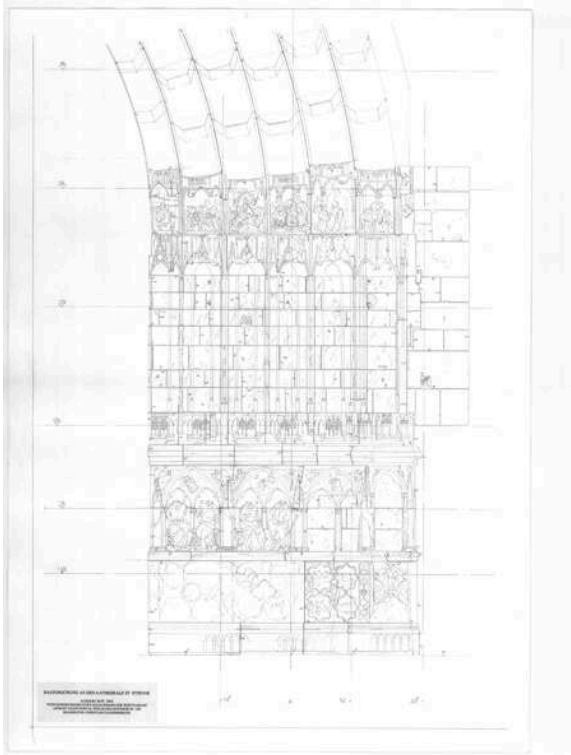
Auxerre, cathédrale Saint-Étienne, façade ouest - portail central, ébrasement sud (dessin H. Hansen - université de Stuttgart).
