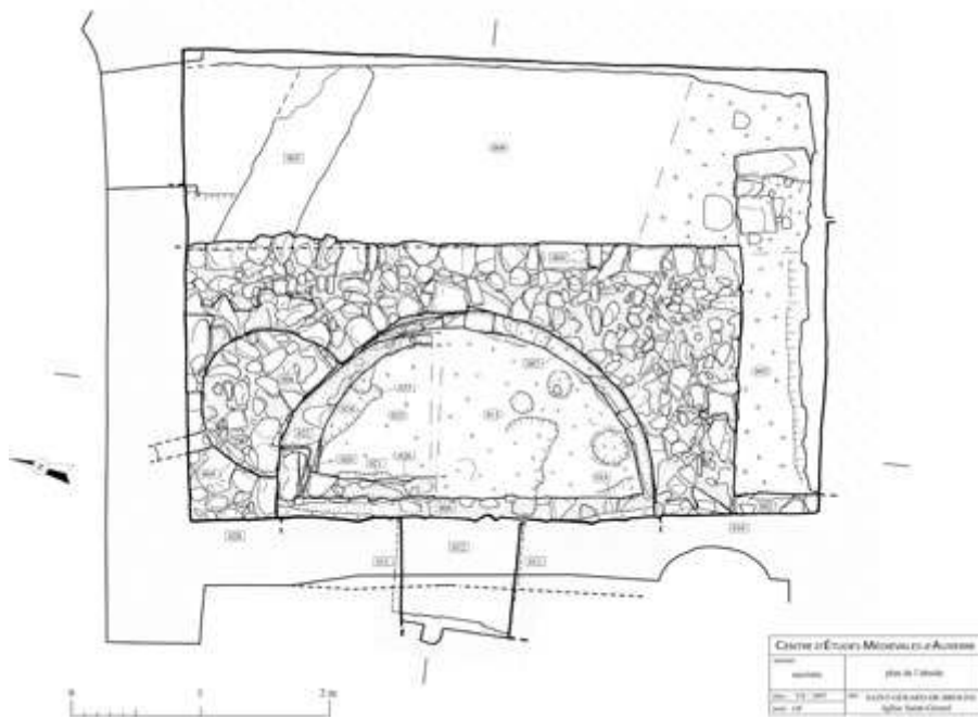
Fig. 2 - Saint-Gérard de Brogne. Plan de l'absidiole (Cliché CEM, G. Fèvre, 2007).
