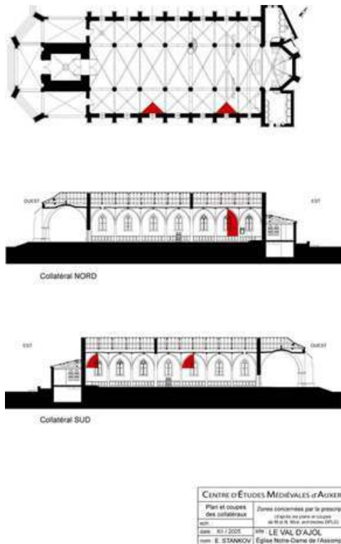
Le Val d'Ajol, église Notre-Dame de l'Assomption. Plan et coupes des collatéraux, zones concernées par la prescription (cliché CEM, XII/2005)
