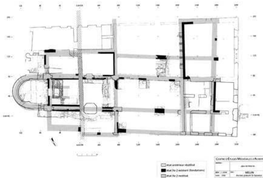
Fig. 1 – Melun, ancien prieuré Saint-Sauveur. Plan de l'état Xe siècle (CEM).
