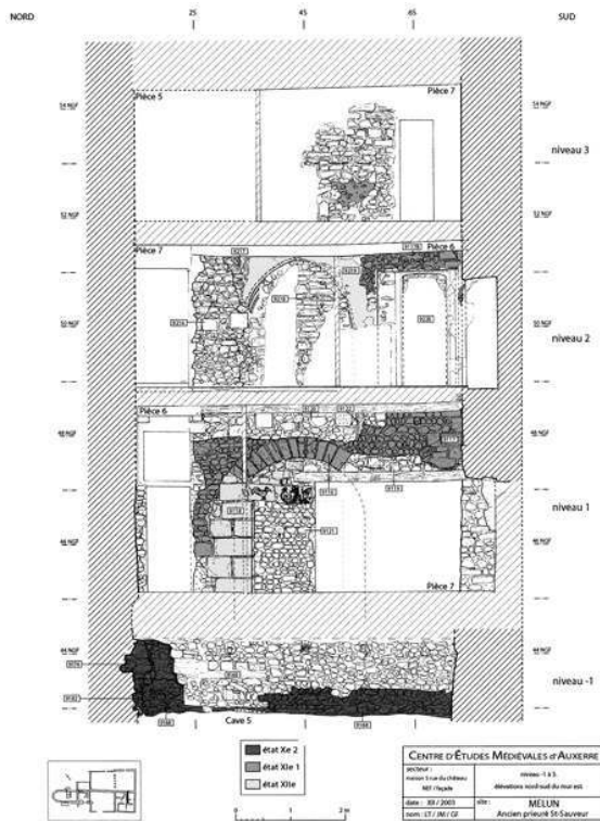
Fig.2 – Melun, ancien prieuré Saint-Sauveur, maison au 5 rue du Château. Nef/façade, élévation N/S du mur est (CEM).
