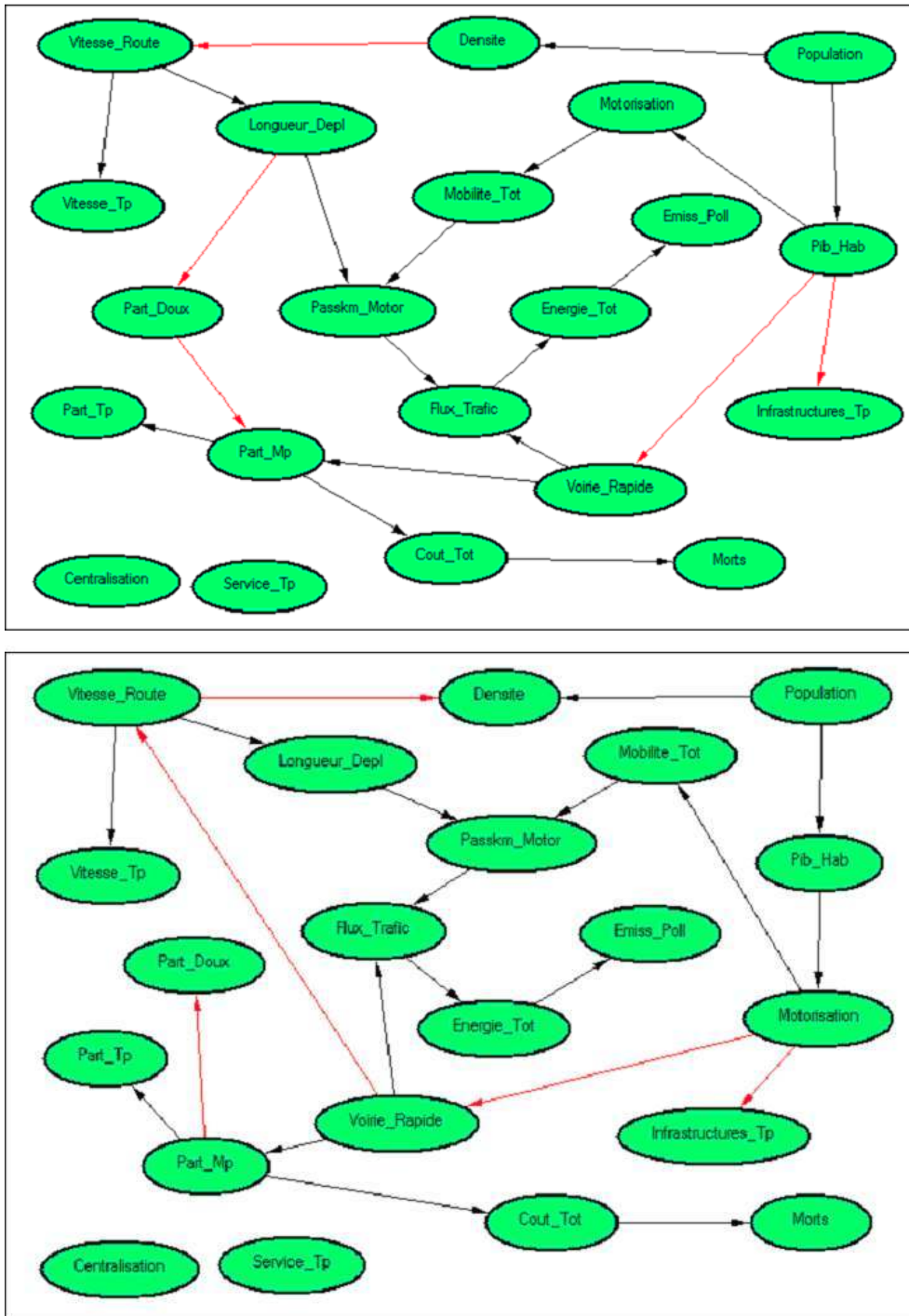
Figure 5 – Les deux réseaux bayésiens générés à partir des 21 variables
