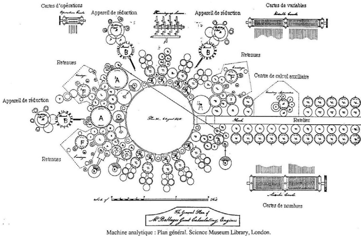
Machine analytique : Plan général. Science Museum Library, London.
