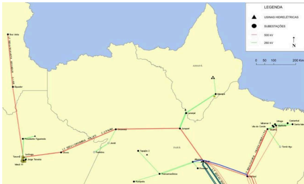
Figura 2 - Sistemas de transmissão compreendidos pelo "linhão de Tucuruí"
