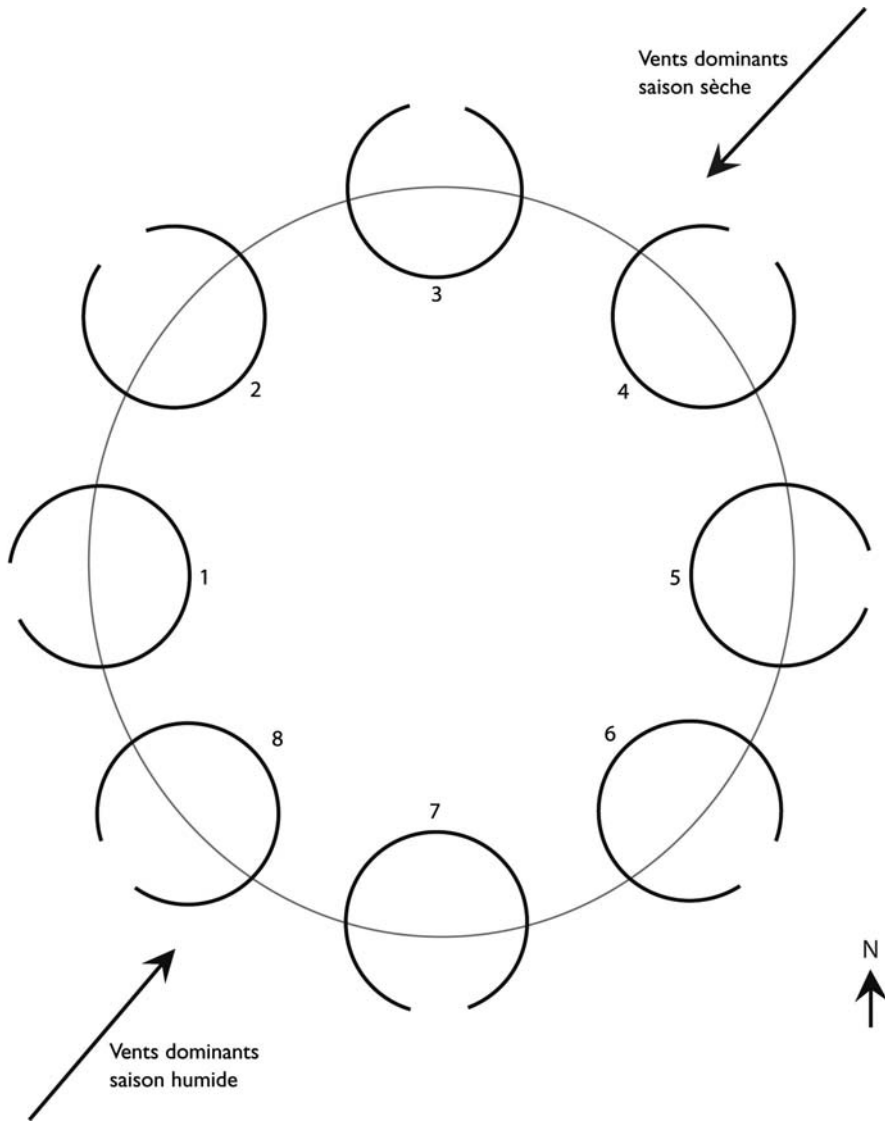
Fig. 4 Orientations possibles de la tente
