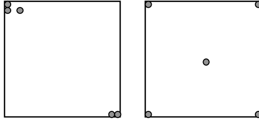
Figure 1. Motifs de 5 points dans un carré maximisant l'étendue (à gauche) et l'étalement-régularité (à droite), définie comme la distance minimale entre deux points du motif
