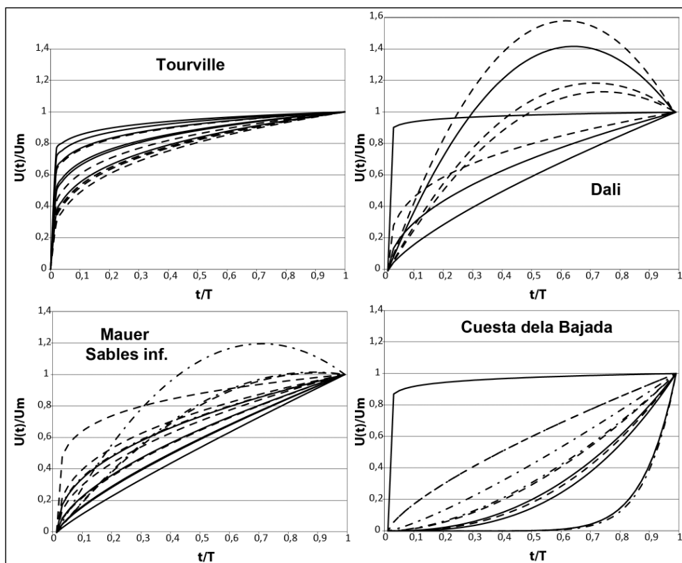
Fig. 4 : Cinétiques d'incorporation de l'uranium modélisées pour les différents tissus des dents provenant des différents gisements considérés. Email : trait continu, dentine : pointillé régulier, cément : pointillé irrégulier. Fig. 4: U-uptake kinetics modeled for all the dental tissues of the present study. Enamel: continuous line, dentine: regularly dotted line, cement: irregularly dotted line.
