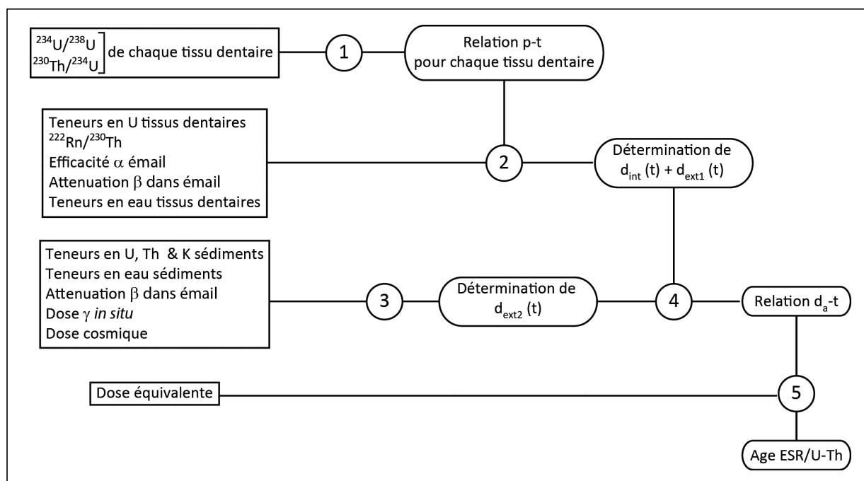
Fig. 3 : Illustration schématique de l'obtention d'un âge couplé ESR/U-Th.
