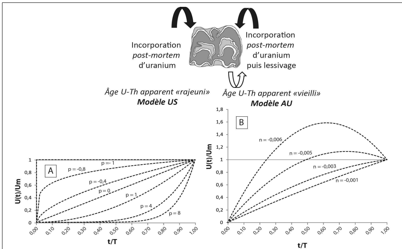
Fig. 2 : Évolution de la teneur relative en uranium dans un tissu paléontologique donné en fonction du temps écoulé par rapport à l'âge pour différents paramètres d'incorporation.
