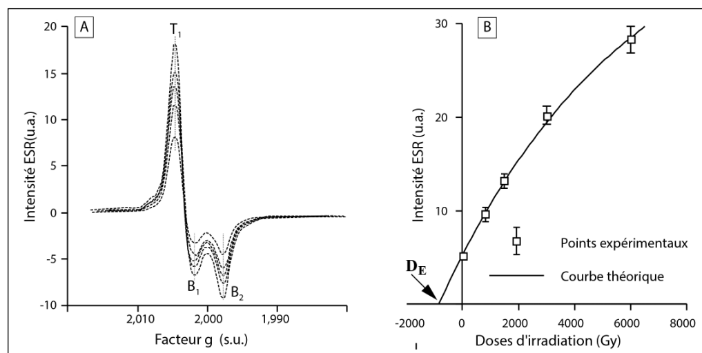
Fig. 1 : Évolution de l'intensité du signal ESR d'un échantillon d'émail dentaire en fonction de doses d'irradiation ajoutées croissantes (A) et courbe de croissance intensité ESR/dose ajoutée pour extrapolation de la paléodose D_E (B).
