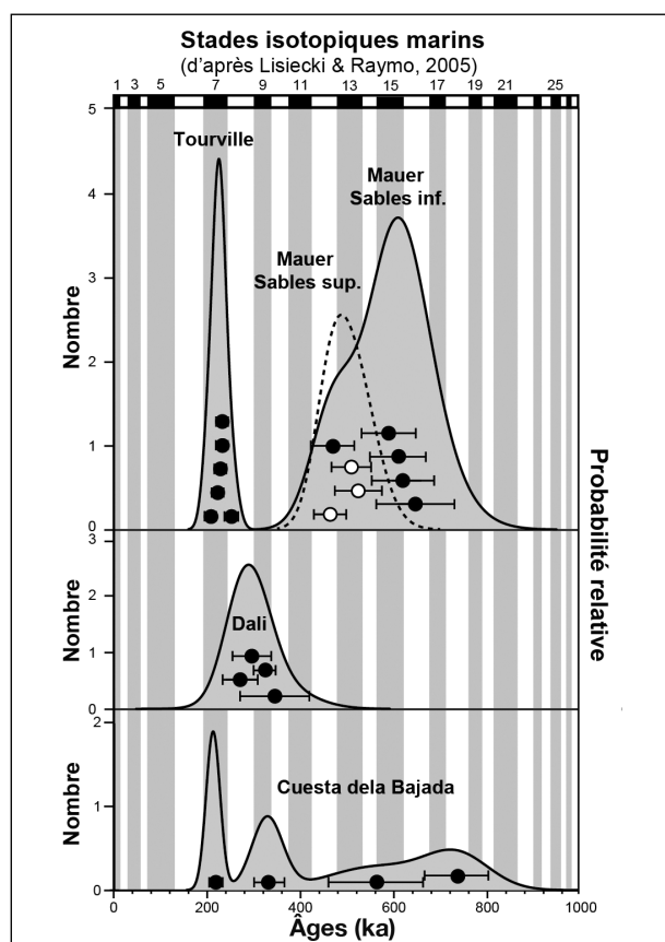
Fig. 5 : Ages ESR/U-Th obtenus sur les échantillons de dents provenant des différents gisements considérés.
