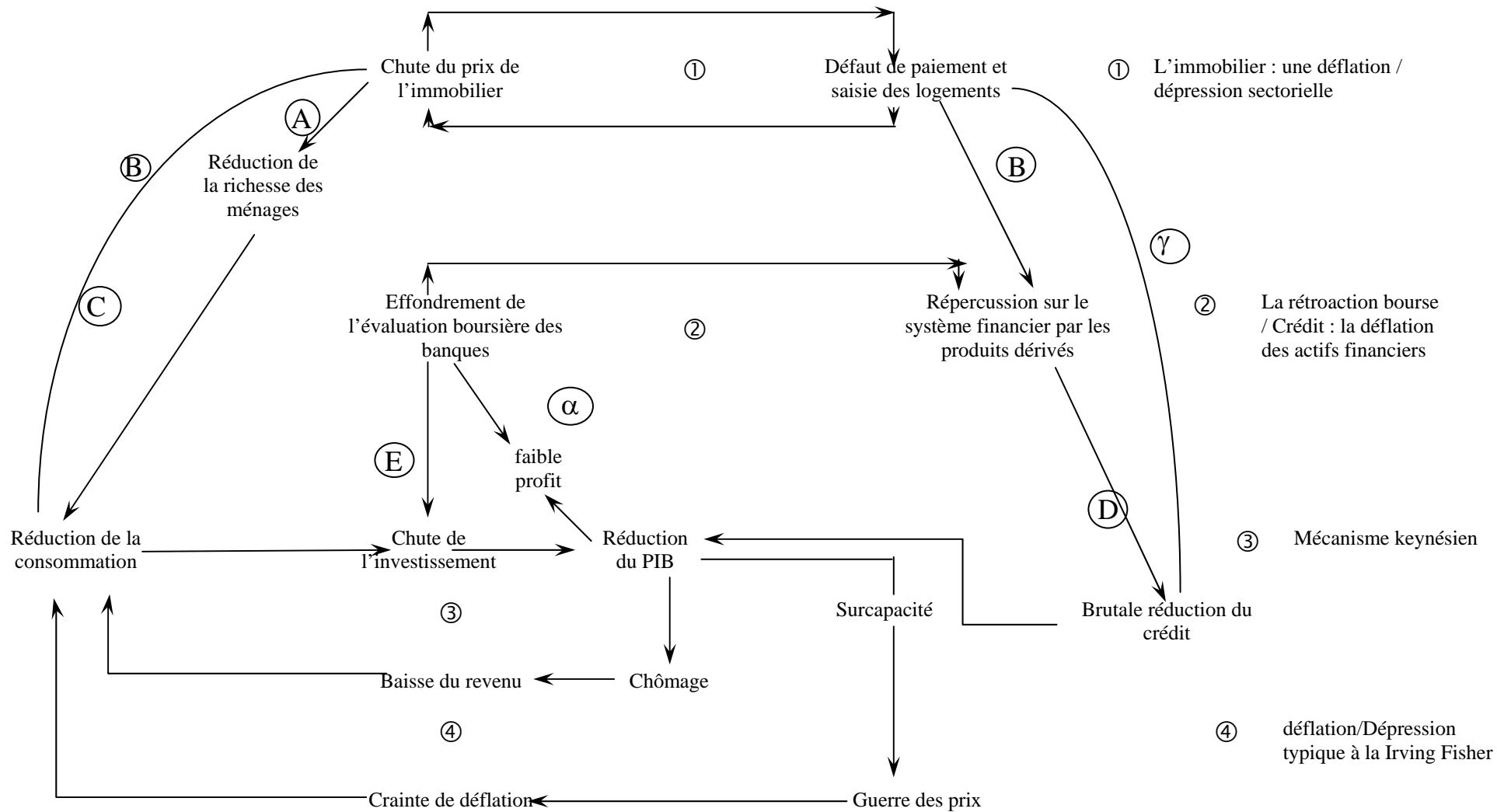
Figure 12 – L’auto-renforcement de trois boucles “déflation – dépression” à la Irving FISHER et ajustement sous la contrainte de crédit
