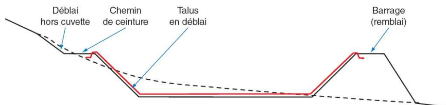
Figure 1 : Principe de la conception en déblai-remblai d'une retenue d'altitude avec une étanchéité d'ensemble de la cuvette avec géomembrane
