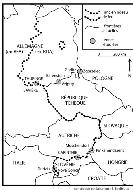
Figure 1 : L'ancien Rideau de fer et localisation des zones étudiées
