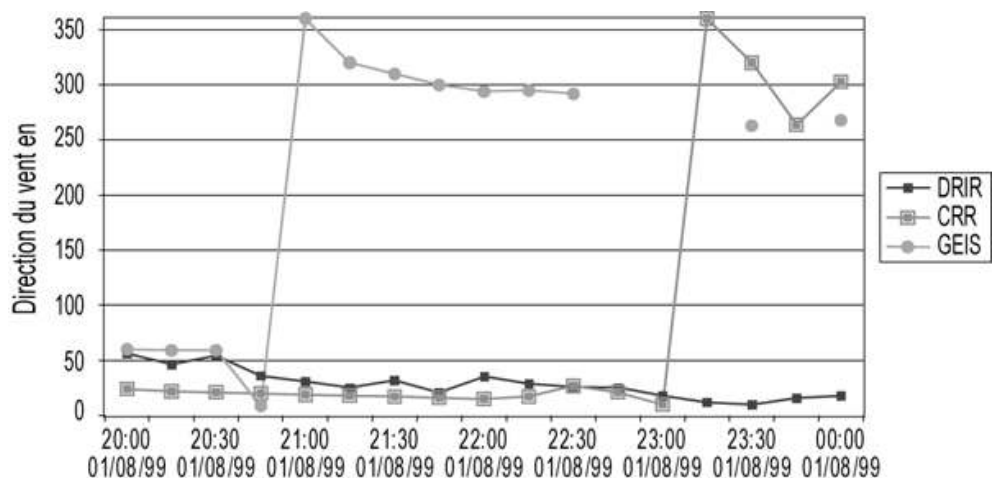
Figure 17 : Direction du vent sur 3 sites entre 20 h et 0 h TU.
