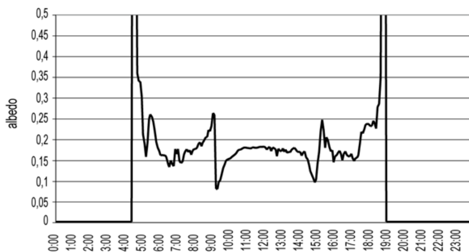
Figure 6 : Albedo le 13 août 1999 sur le site de l'avenue de Gaulle à 10 m de hauteur.
